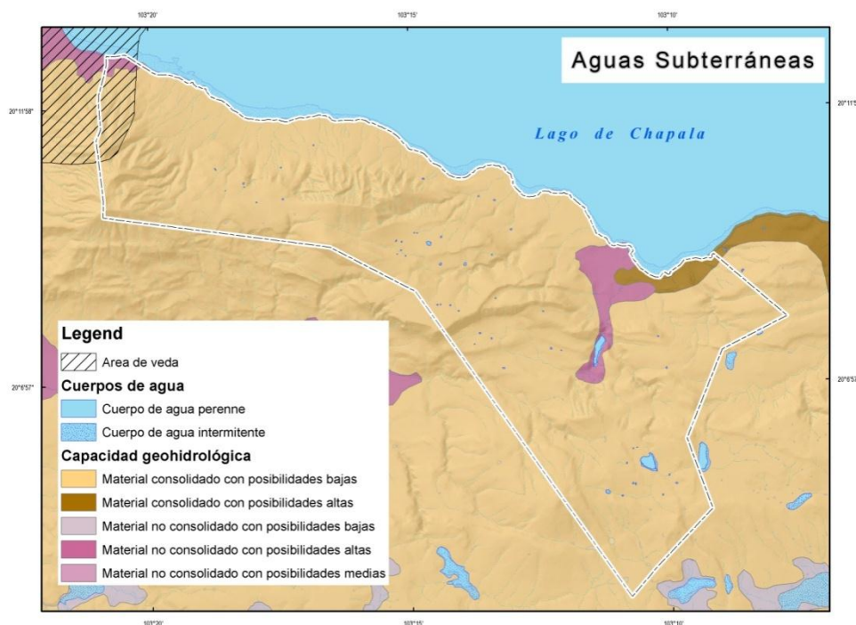
Ilustración 1 Secuencia geológicas con posibilidades de albergar acuíferos importantes.
