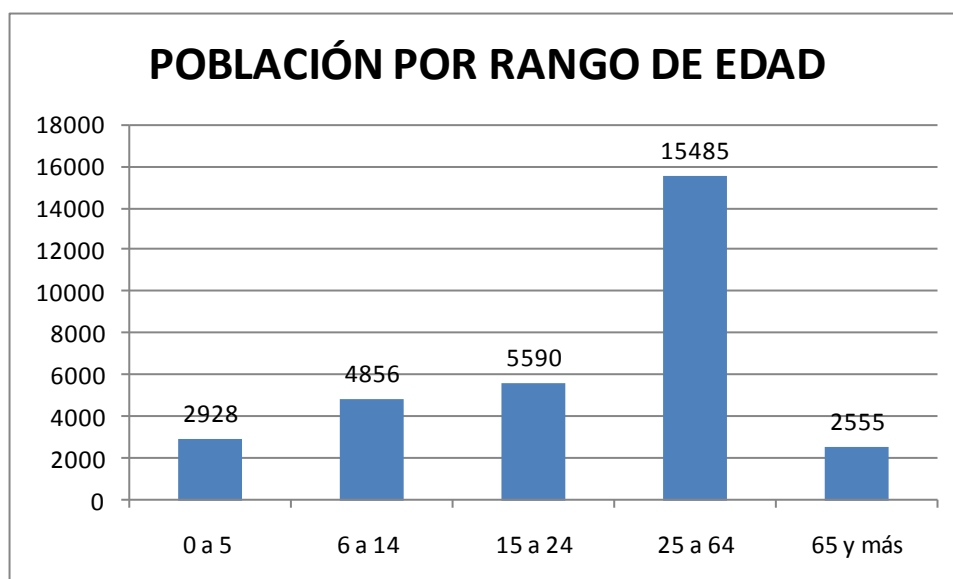
Gráfica 12. Población por rango de edad. Subdistrito Urbano 2 “FerrocarriI” del Distrito Urbano 7 “Zona Cruz Del Sur”; Fuente: II Censo de Población y Vivienda 2005. INEGI.
