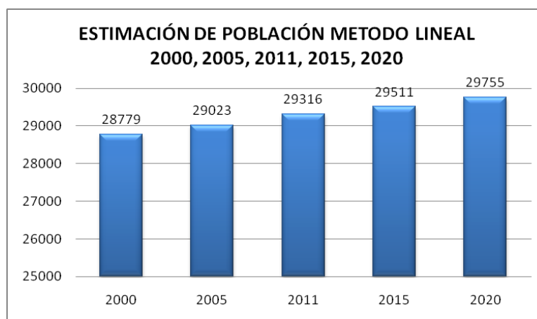
Gráfica 25. Proyección demográfica aplicando el método lineal.
