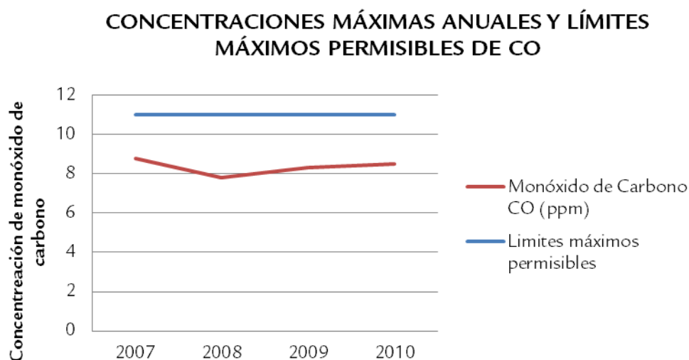
Gráfica 25. Concentraciones máximas anuales de CO y límites máximos permisibles.
