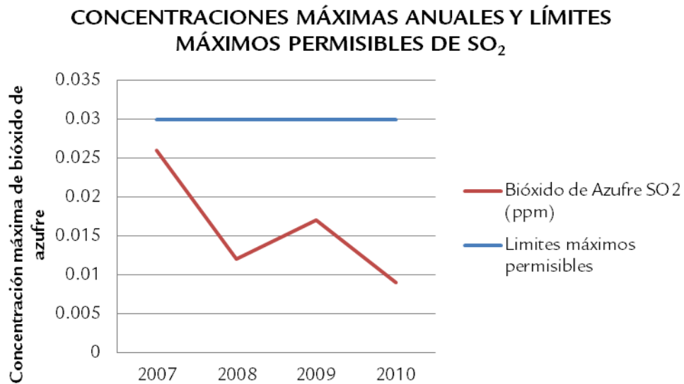
Gráfica 27. Concentraciones máximas anuales de SO 2 y límites máximos permisibles.
