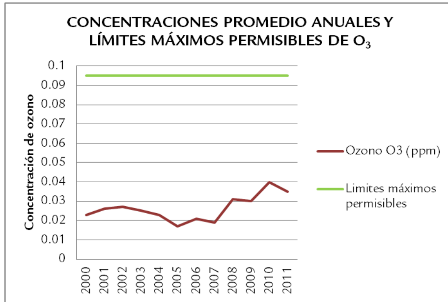
Gráfica 20. Concentraciones promedio anuales y límites máximos permisibles de O 3 Fuente: Elaboración propia con datos de SEMADET, 2014.
