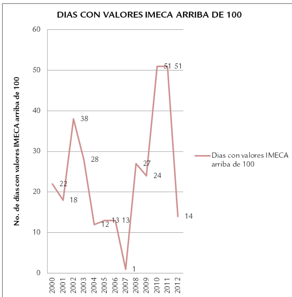
Gráfica 31. Días al año que sobrepasaron los 100 IMECAS en la estación Vallarta.
