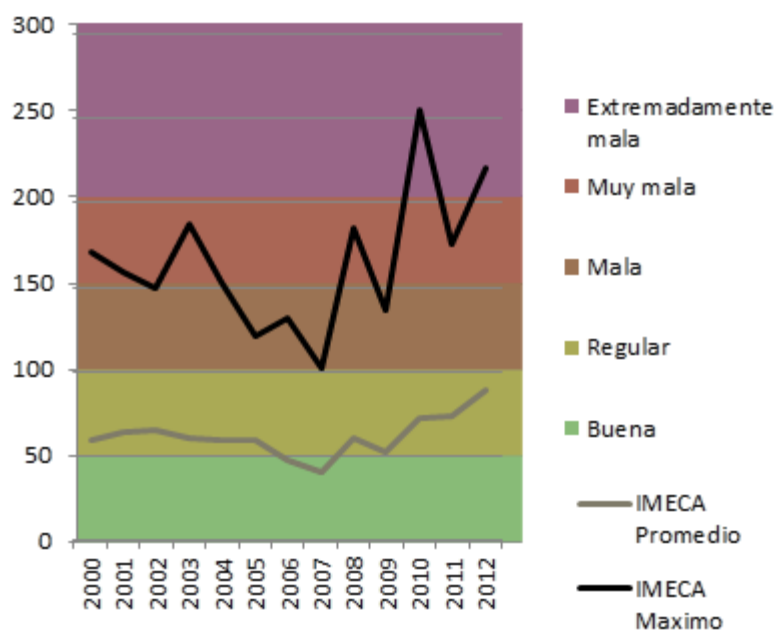
Gráfica 30. IMECAS máximos y promedio anuales.
