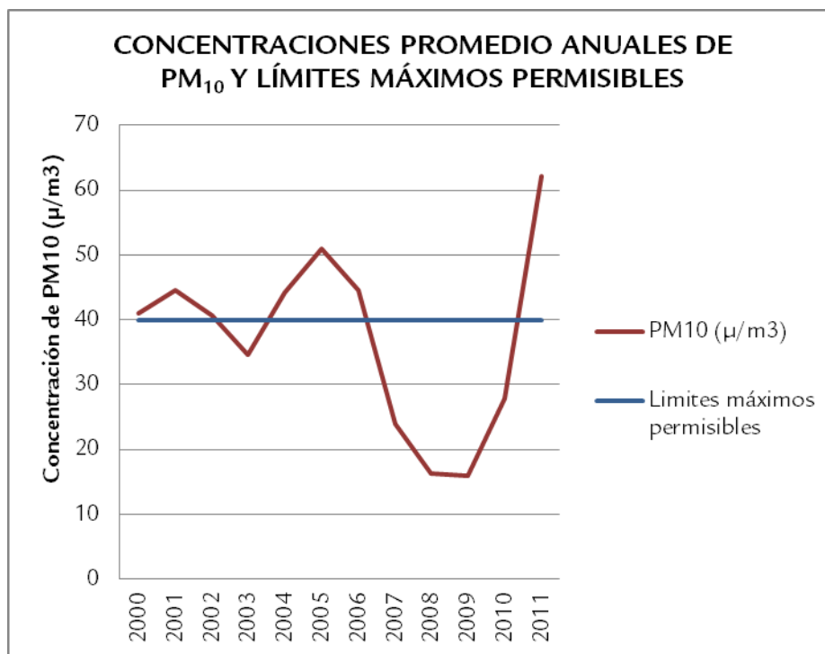
Gráfica 28. Concentraciones promedio anuales de PM_{10} y límites máximos permisibles.
