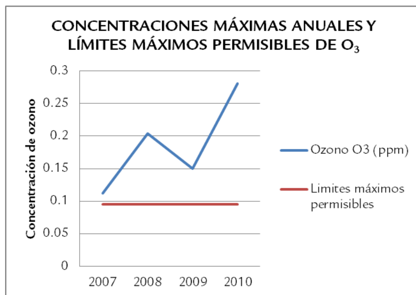
Gráfica 21. Concentraciones máximas registradas por año y límites máximos permisibles de O 3 . Fuente: Elaboración propia con datos de SEMADET, 2014.
