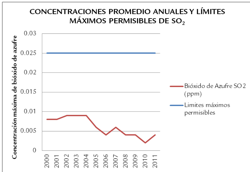
Gráfica 26. Concentraciones promedio anuales de \text{SO}_2 y límites máximos permisibles.
