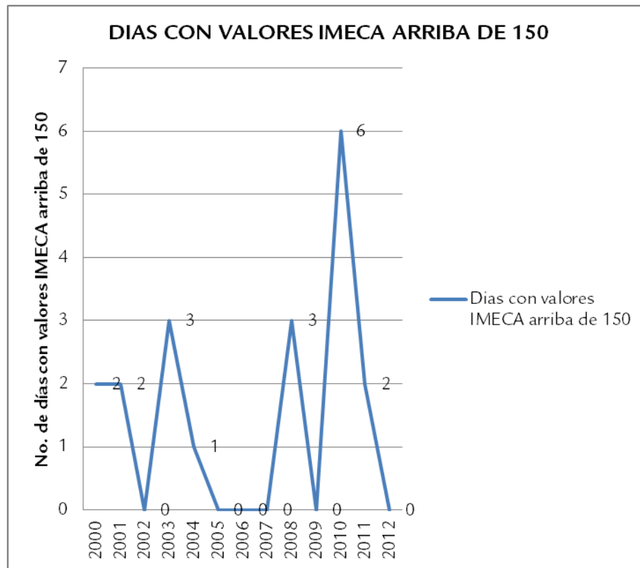
Gráfica 32. Días al año que se rebasaron los 150 IMECAS en la estación Vallarta.
