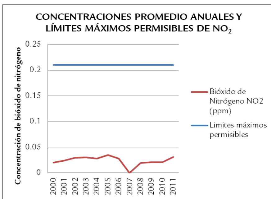
Gráfica 22. Concentraciones promedio anuales y límites máximos permisibles de \text{NO}_2 .
