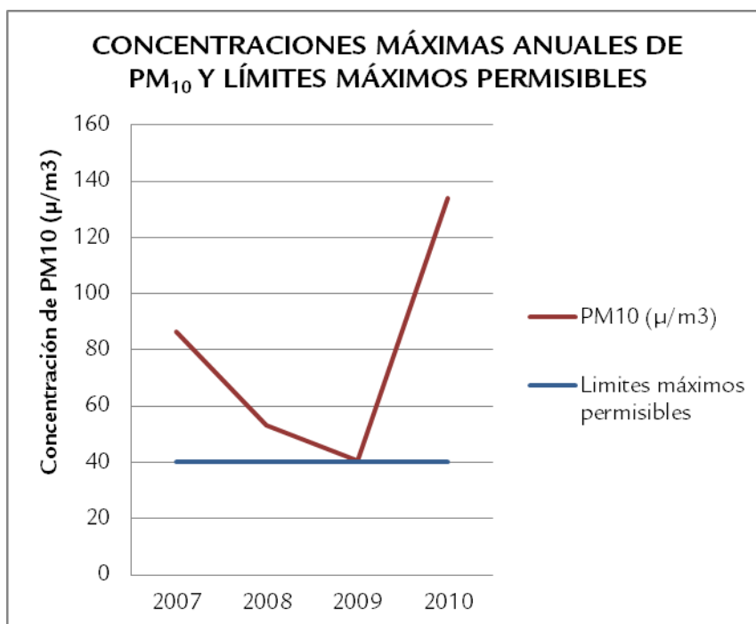
Gráfica 29. Concentraciones máximas anuales de PM 10 y límites máximos permisibles.
