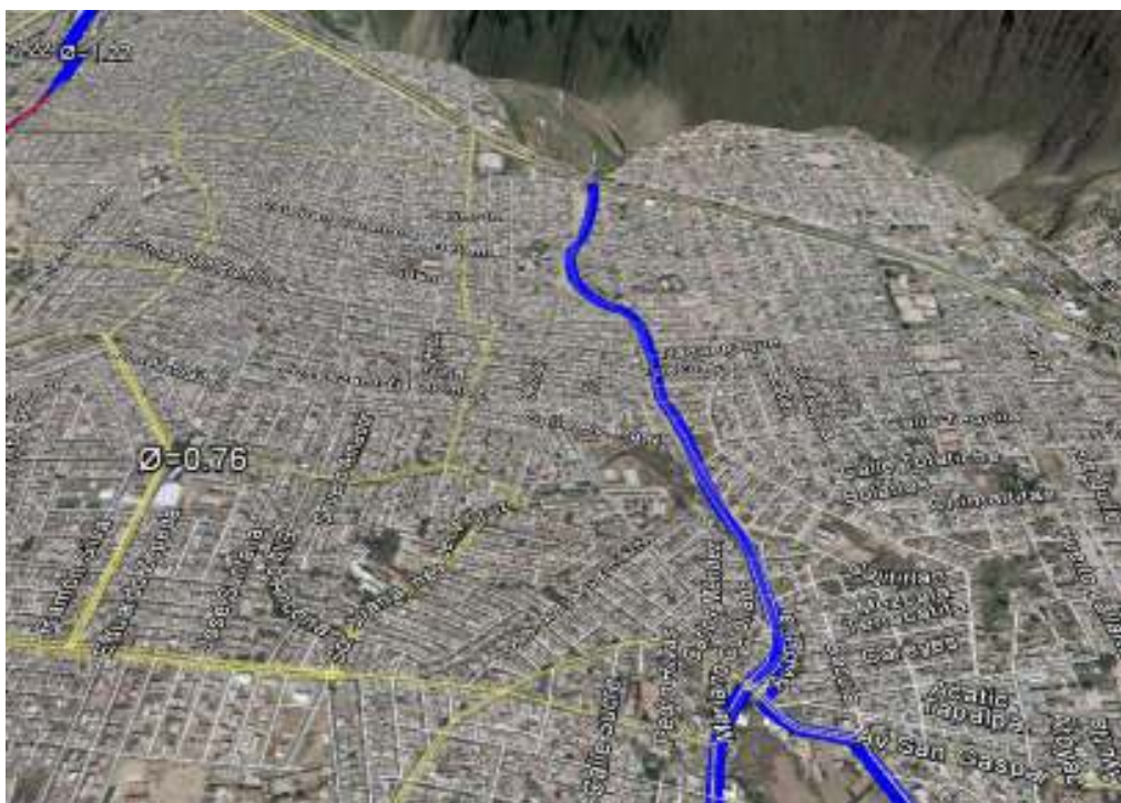
Ilustración 15. Localización de colectores en el subdistrito. Fuente: Elaboración propia a partir de datos de CEA y SIAPA.
