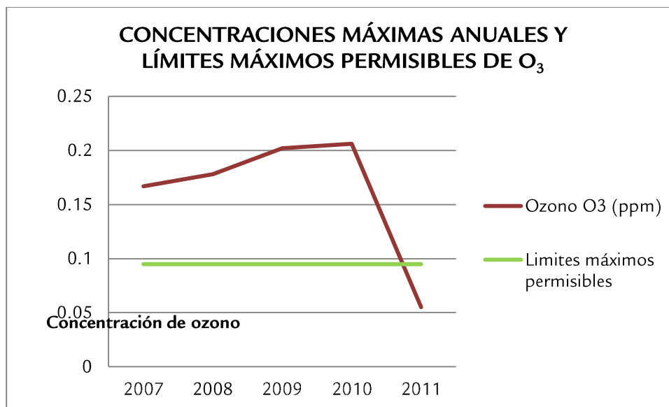
Gráfica 21. Concentraciones máximas anuales de O 3 y límites máximos permisibles.
