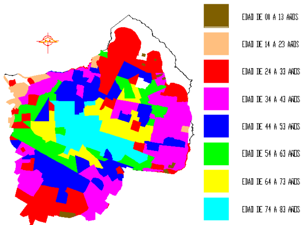
Ilustración 12. Edades de tuberías de agua potable dentro del municipio de Guadalajara. Fuente: SIAPA
