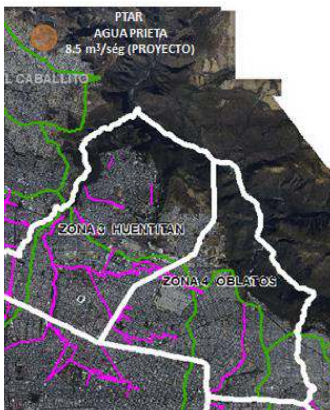
Ilustración 16. Localización del distrito Zona 4 “Oblatos” con respecto a las cuencas hidrológicas y la PTAR Agua Prieta. Fuente: Elaboración propia a partir de datos de CEA y SIAPA.
