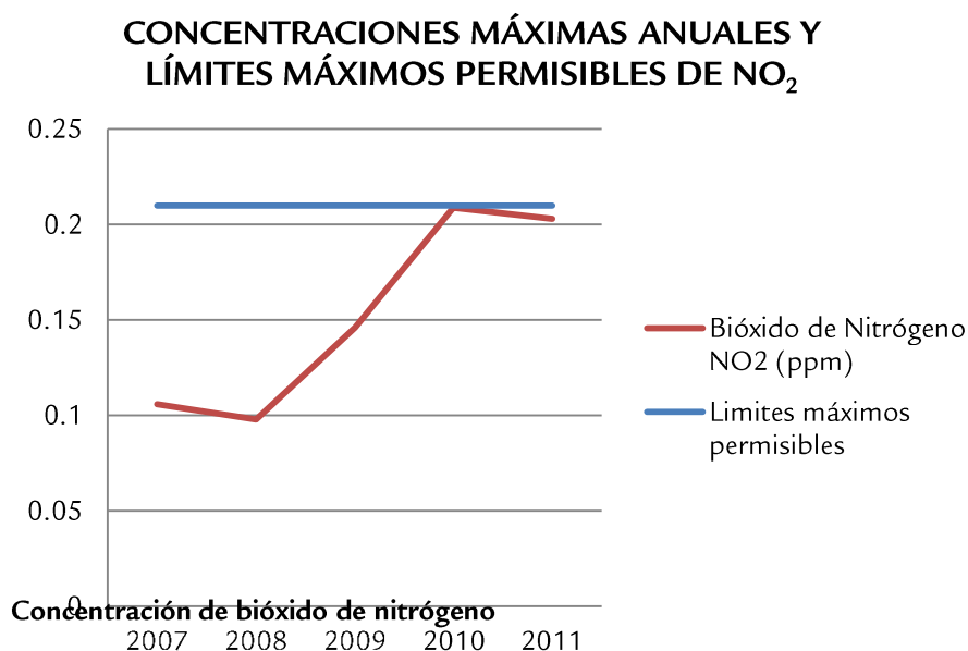
Gráfica 23. Concentraciones máximas anuales de NO 2 y límites máximos permisibles
