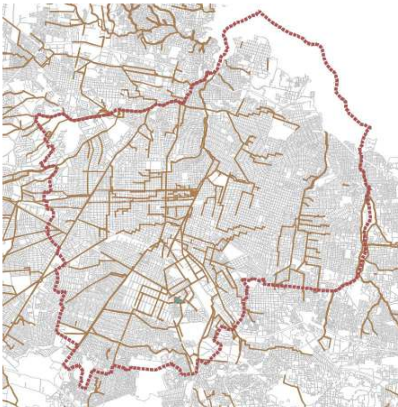
Ilustración 14. Colectores principales dentro del municipio de Guadalajara.
